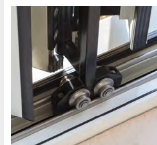
Bottom Roller
